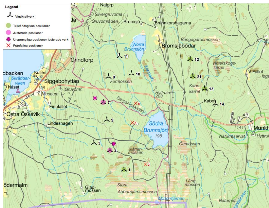
Bild 1 – Justerade verkspositioner.
